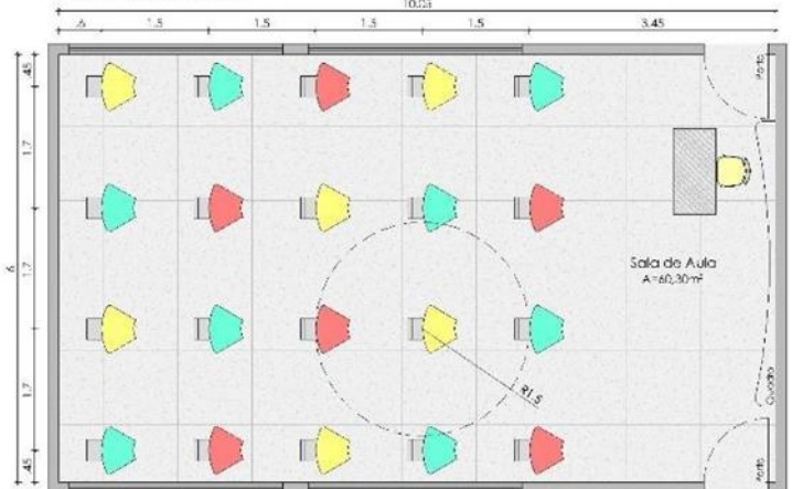
PLANTA BAIXA DA SALA DE AULA - 20 crianças ESCALA 1/50
