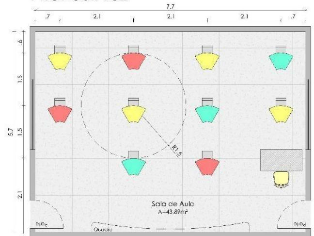
PLANTA BAIXA DA SALA DE AULA - 10 crianças ESCALA 1/50
