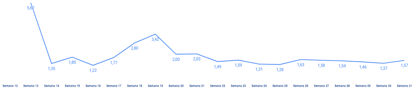
Figura 6. R0 suavizado por semana epidemiológica em Palmas-TO, 2020.
