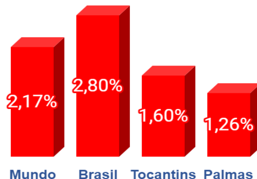
Gráfico 4. Letalidade dos casos de covid-19, 2020-2021.
