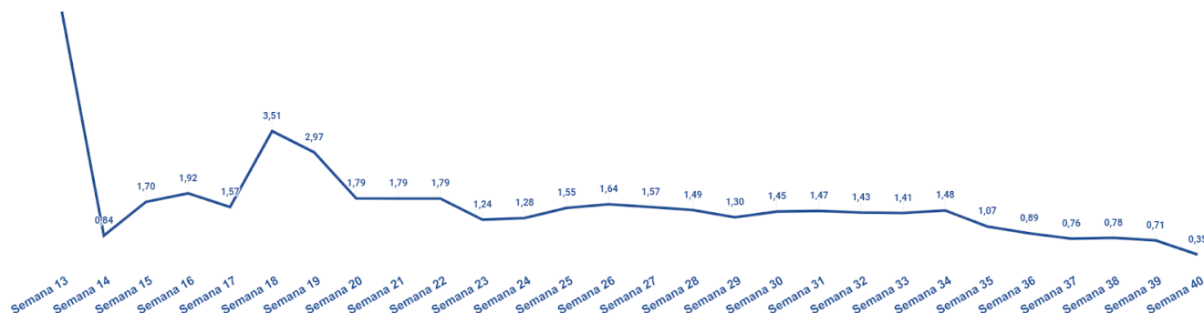
Gráfico 5. R_0^* por semana epidemiológica em Palmas-TO, 2020.
