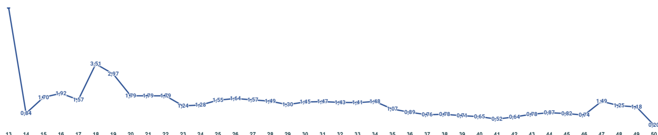
Gráfico 5. Média do R_0^* por semana epidemiológica em Palmas-TO, 2020.
