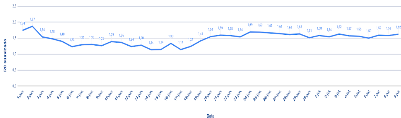
Figura 6. R0 suavizado por dia em Palmas-TO, 2020.
